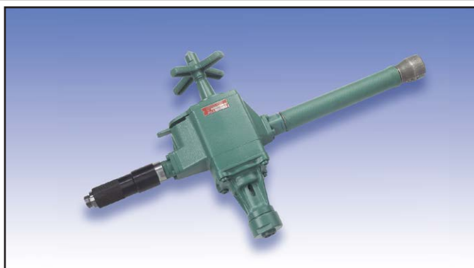
Abb.: Druckluft-Bohrmaschine 2 2089 0030
